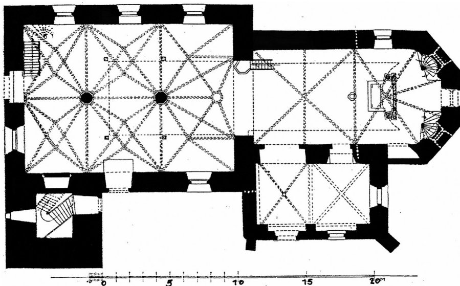
Abb. 2: Kirche Hirschfelde, Grundriss 2008 (nach GURLITT, S. 53), bearbeitet vom Autor
